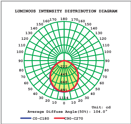
Fotometría - Eficacia: 113 lm/w
